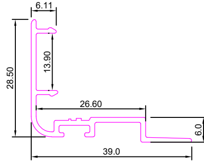
Euro Clip
