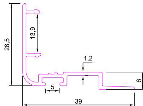
Clip
